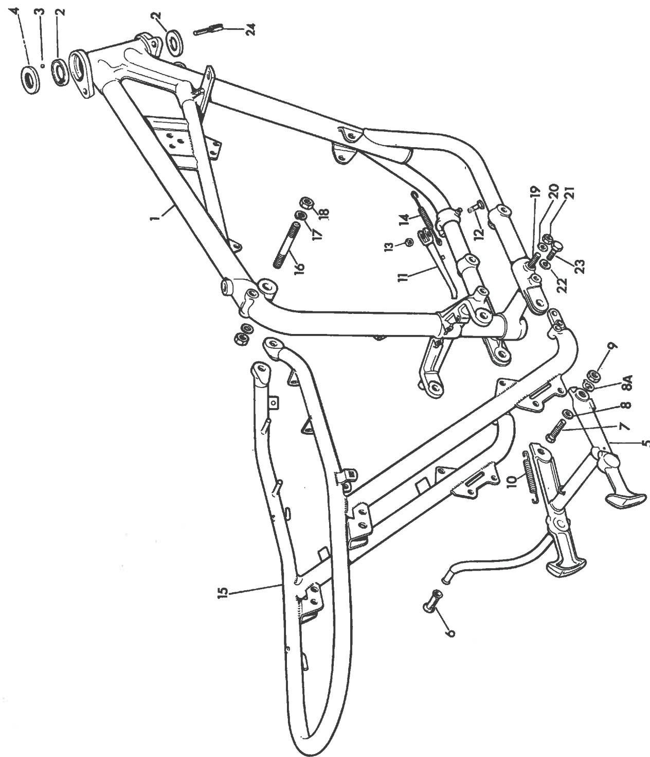
Fig. 12. FRAME
