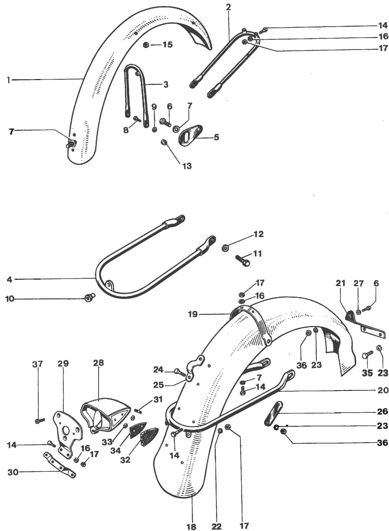
Fig. 26. FENDERS
